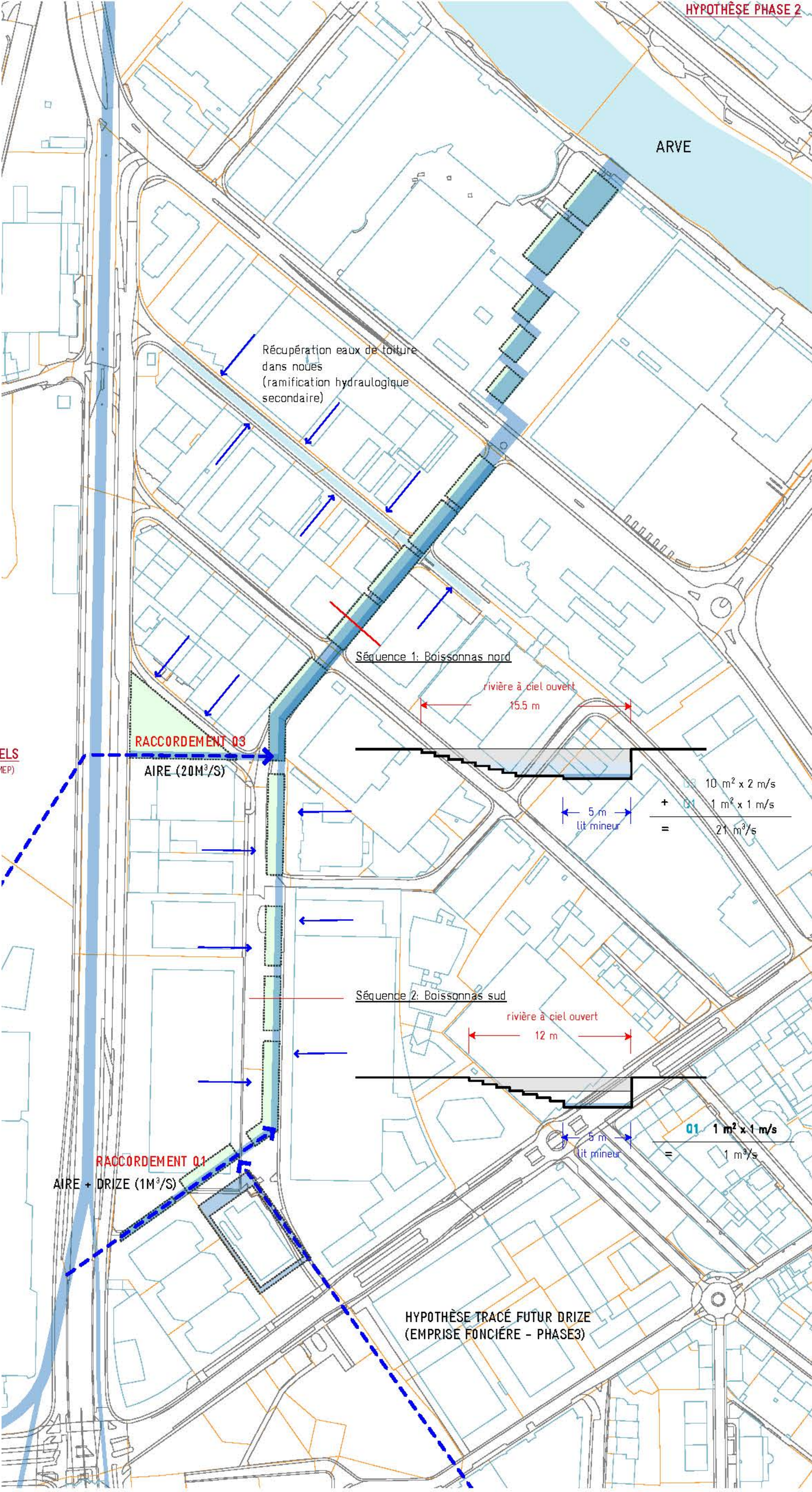
PHASE 1 - AMÉNAGEMENT RUE BOISSONNAS
