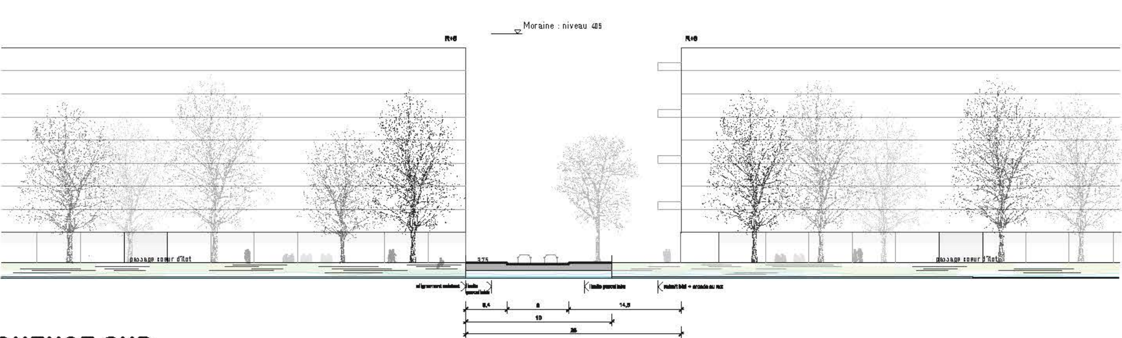
D-D : RUE MARZIANO
