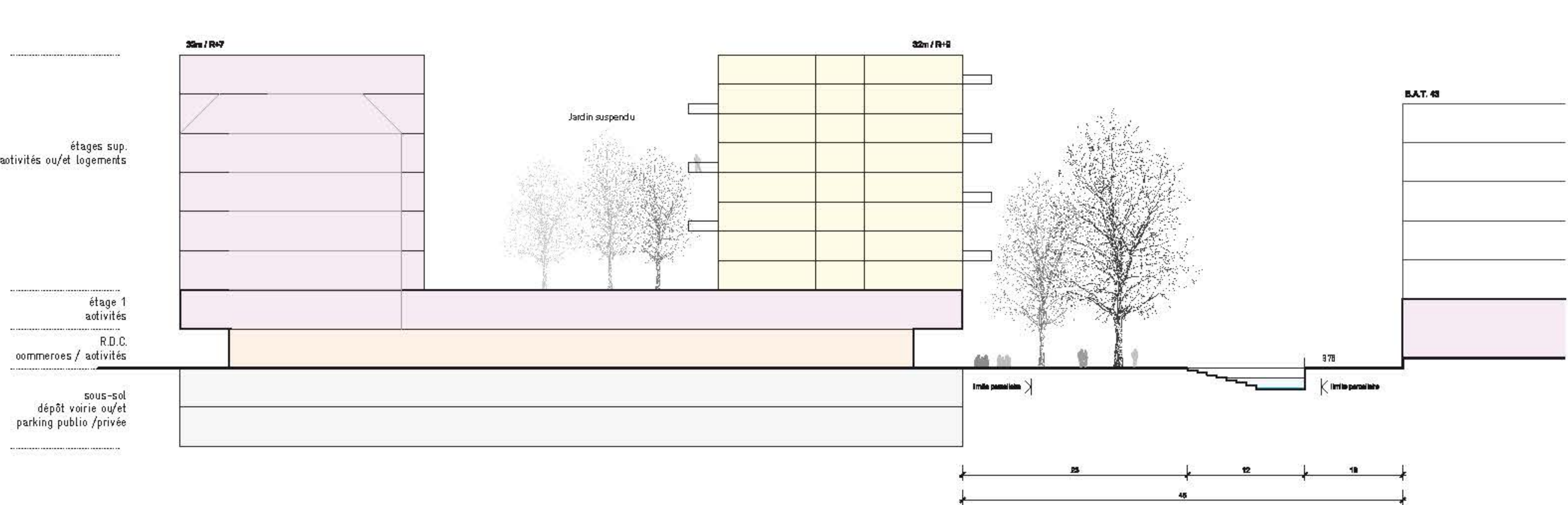
E-E : RUE BOISSONNAS / ROUTE DES JEUNES
