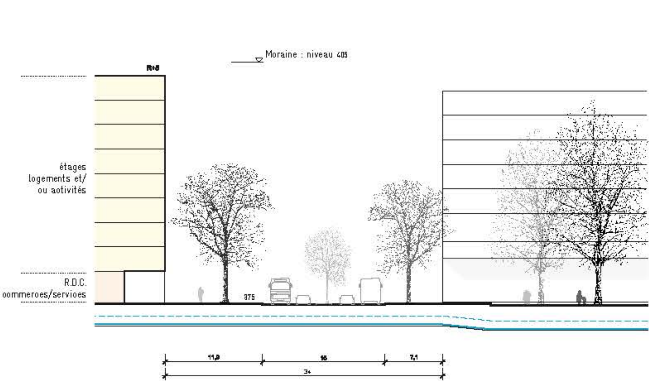
C-C : RUE FRANÇOIS-DUSSAUD
